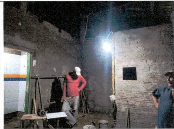
FOTO 14: Elementos estruturais;
