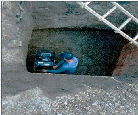
Foto 03: Execução de reforço de solo.
