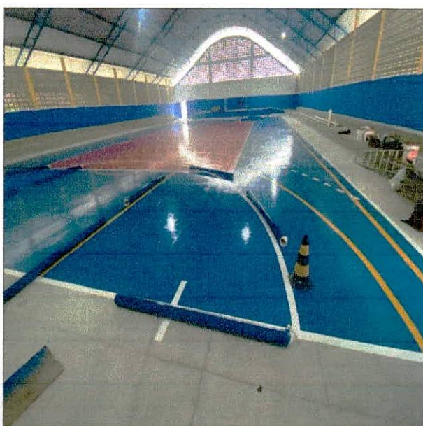
Foto 04: Execução de reparo de alvenarias e recomposição de revestimentos.
