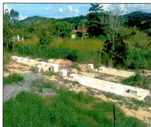
Foto 12: Sistema de destino final de esgotos executado.
