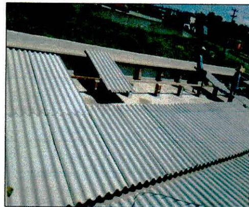
Foto 04: Execução de Coberta.
