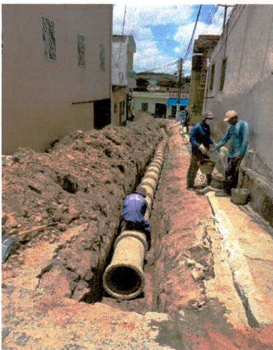
Tubo de concreto simples 400mm
