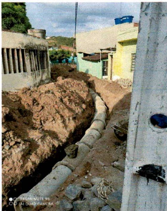
Tubo de concreto simples 400mm
